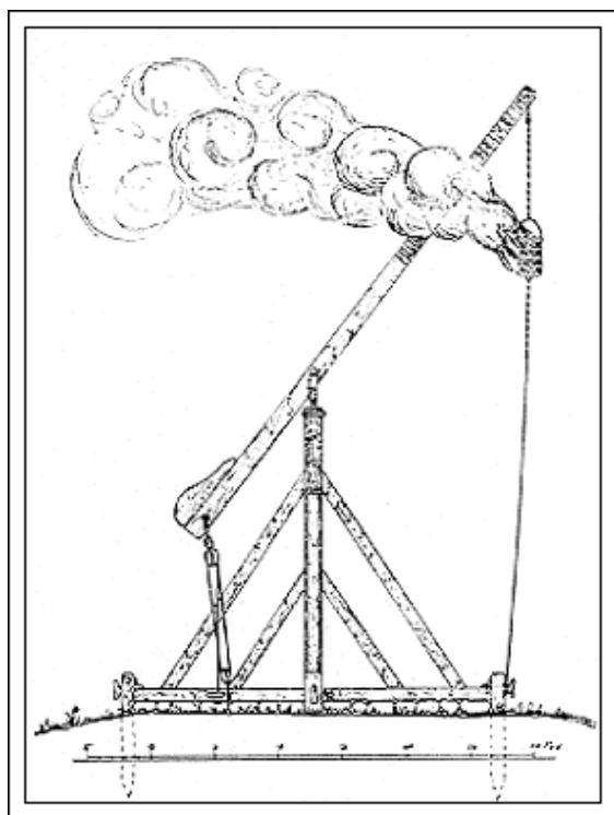
Original konstruktionstegning til vippefyr på Ostebakken. - www.anholt.dk/fyret.htm
